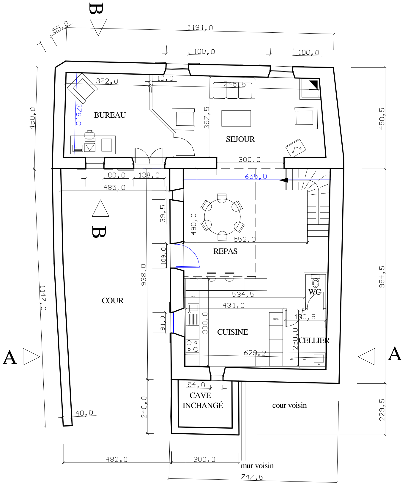
PROJET PLAN Rez de chaussée 1/100
